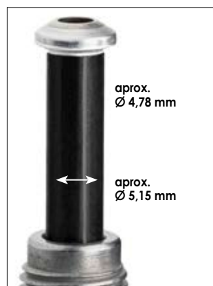
Posicionamiento del conducto para raspar el revestimiento
