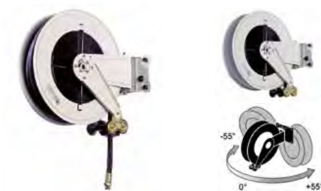
Stainless steel industrial hose reels with ABS shock proof drum. Avvolgitubo industriali in acciaio inox con tamburo in ABS antiurto.
